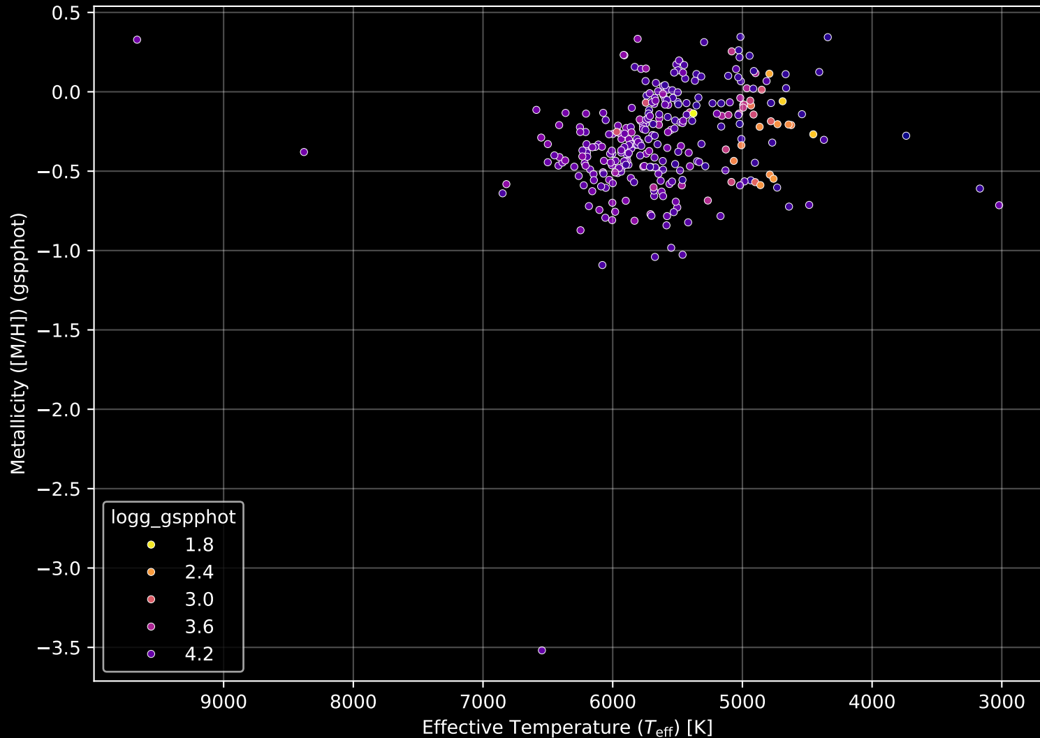
GALAH DR4 Field: [130] Stellar Population Parameters (n= 296)
