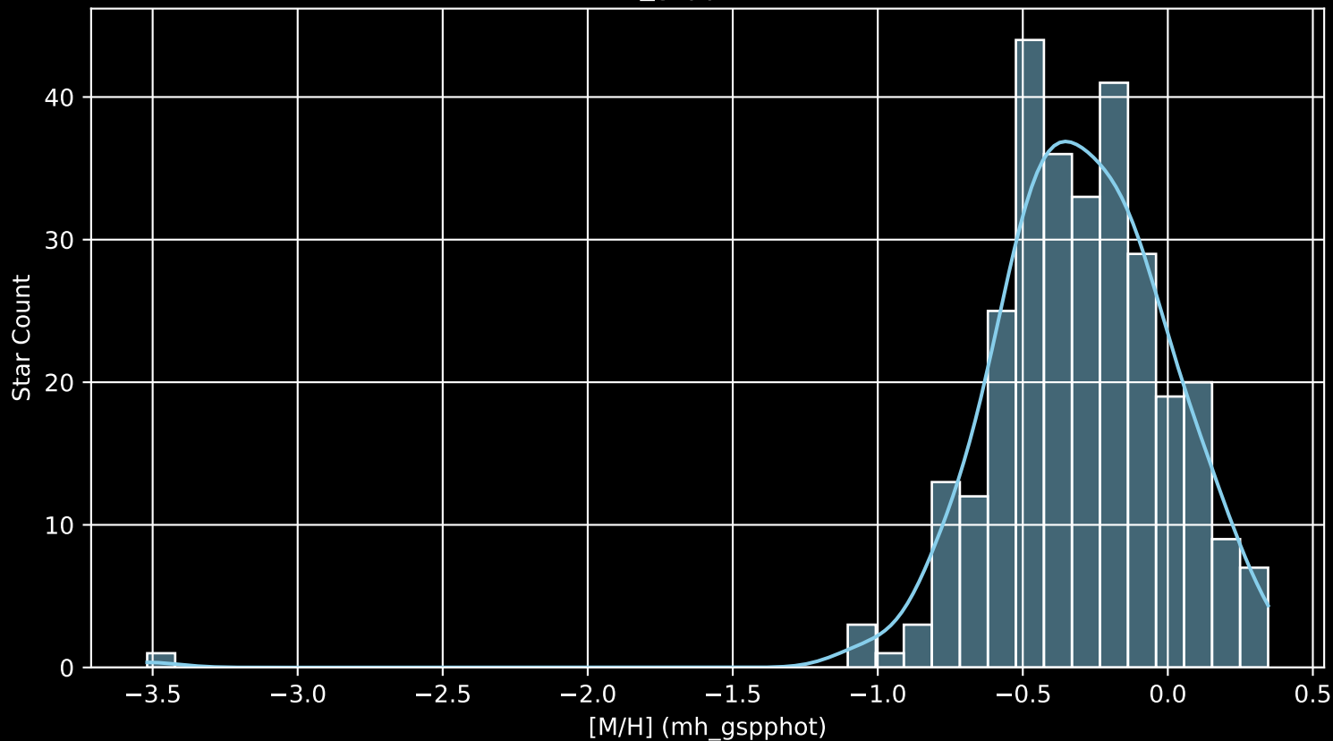
GALAH DR4 Field: [130] [M/H] (mh_gspphot) (n= 296)
