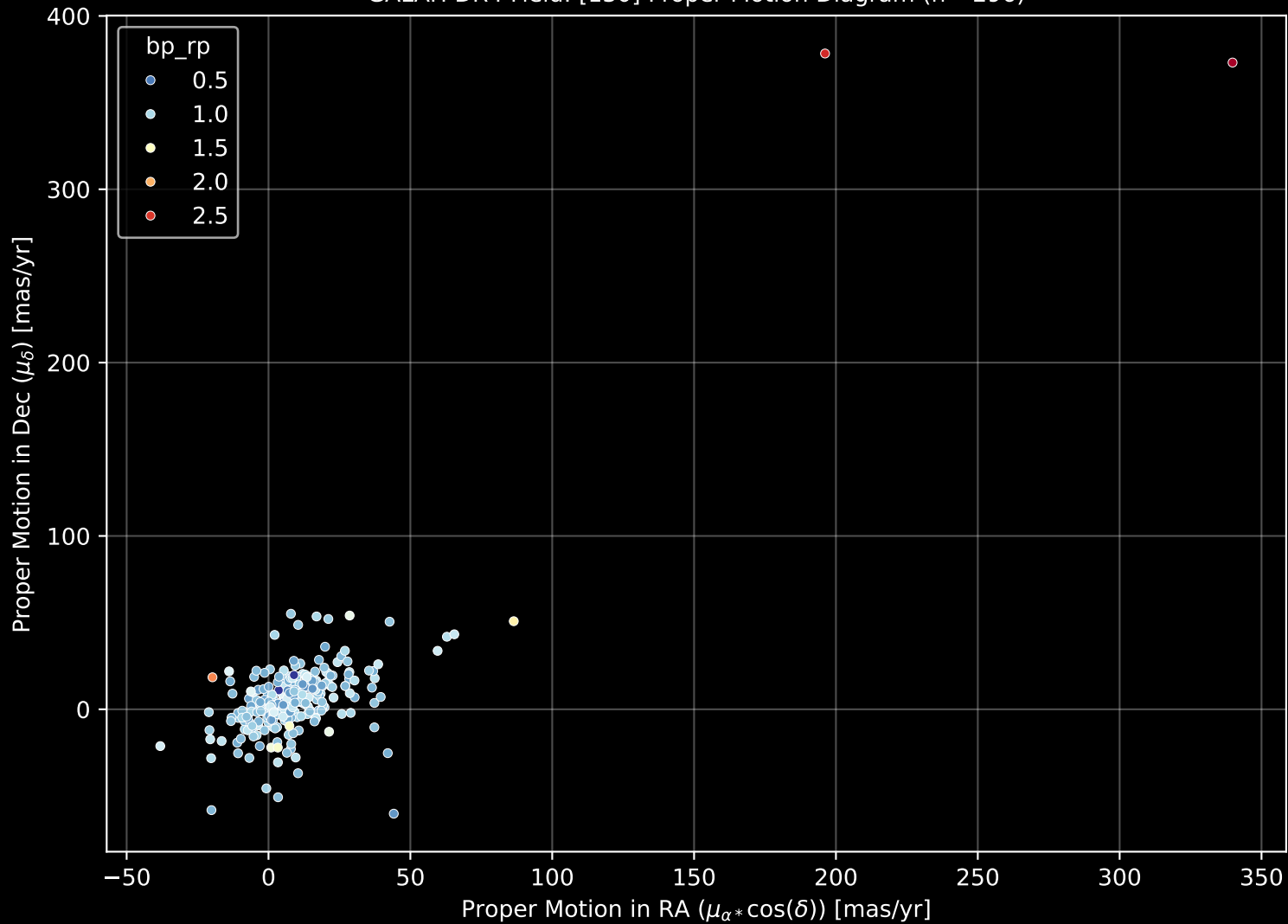
GALAH DR4 Field: [130] Proper Motion Diagram (n= 296)
