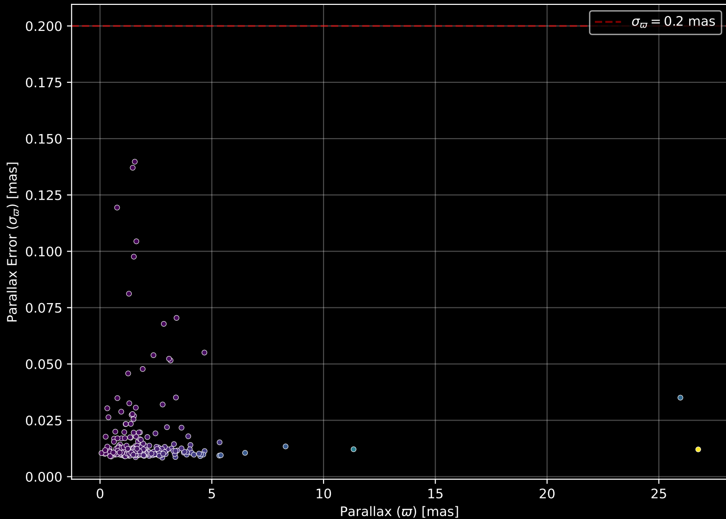
GALAH DR4 Field: [130] Parallax Quality (n= 296)
