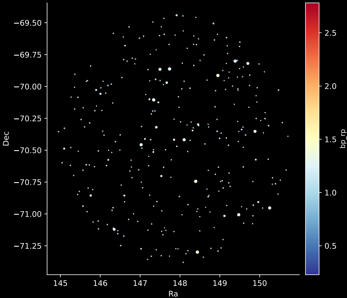
GALAH DR4 Field: [130] Stars: 296
